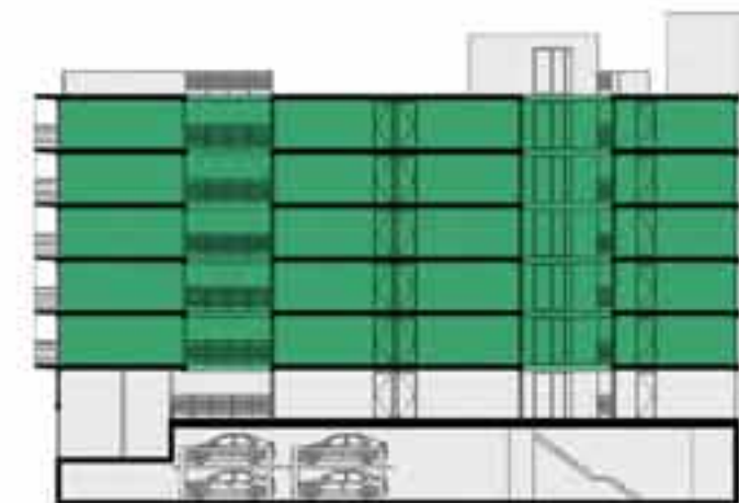
CORTE ESQUEMATICO
