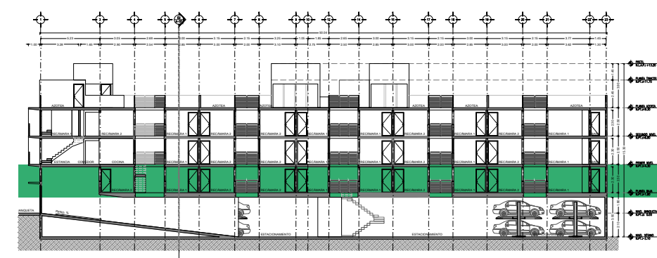
CORTE ESQUEMATICO
