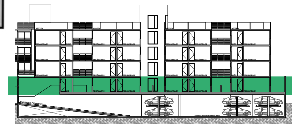
CORTE ESQUEMATICO
