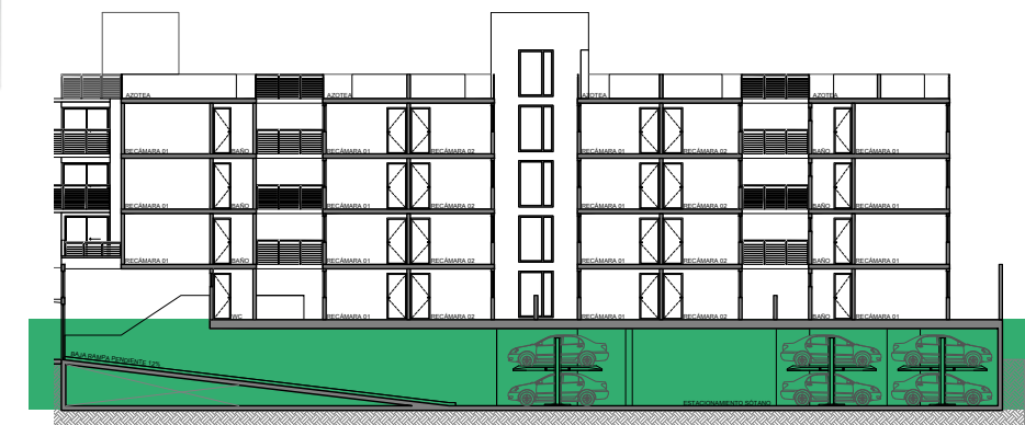
CORTE ESQUEMATICO
