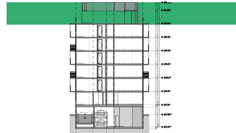
CORTE ESQUEMATICO
