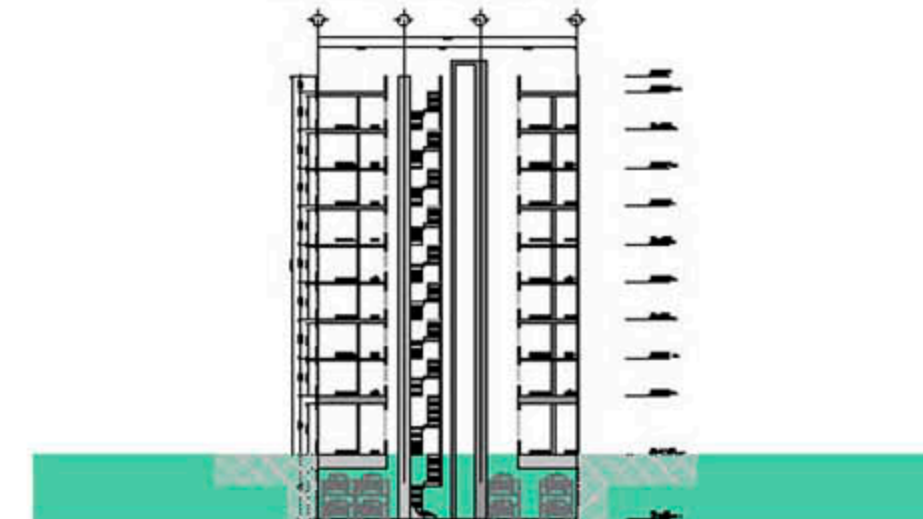
SECCIÓN ESQUEMATICA
