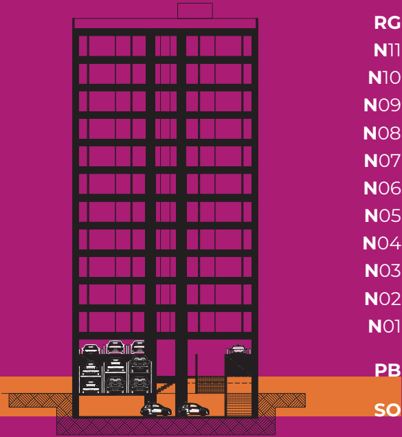
Sección esquemática
