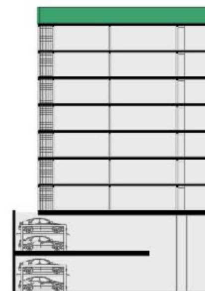
CORTE ESQUEMATICO
