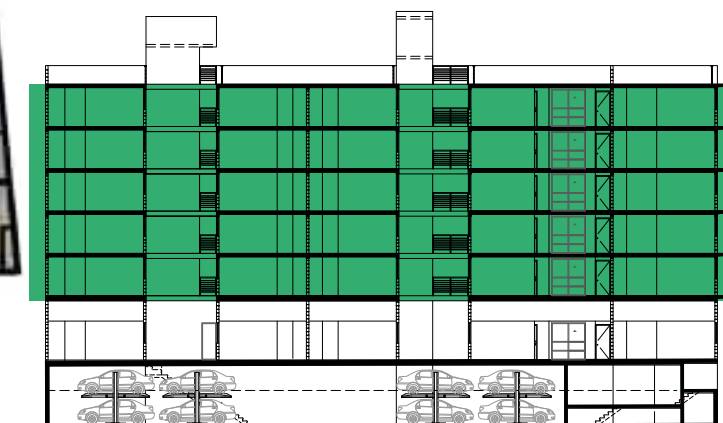
CORTE ESQUEMATICO
