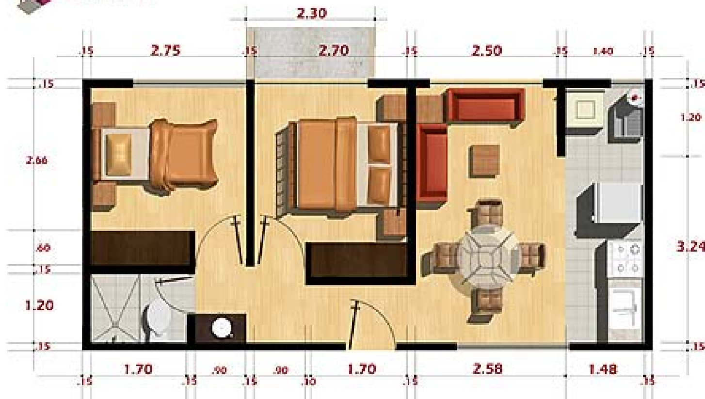
planta ARQUITECTÓNICA
