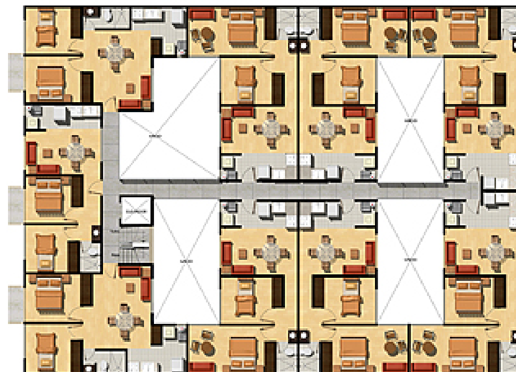
PLANTA TIPO NIVELES 2-6
