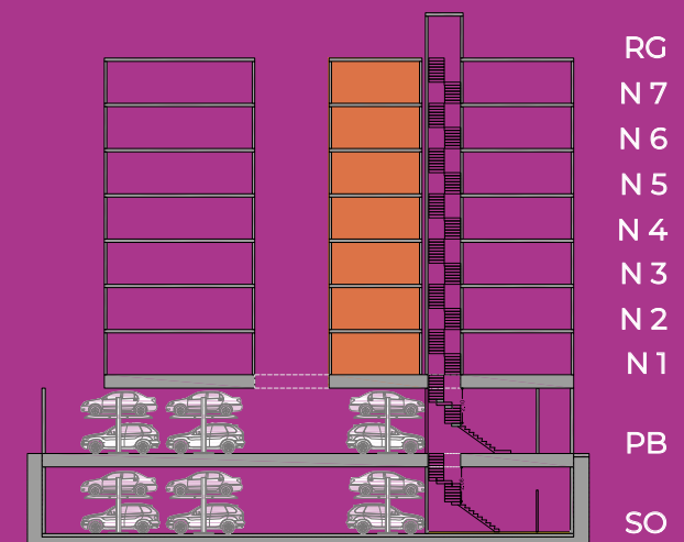
Sección esquemática
