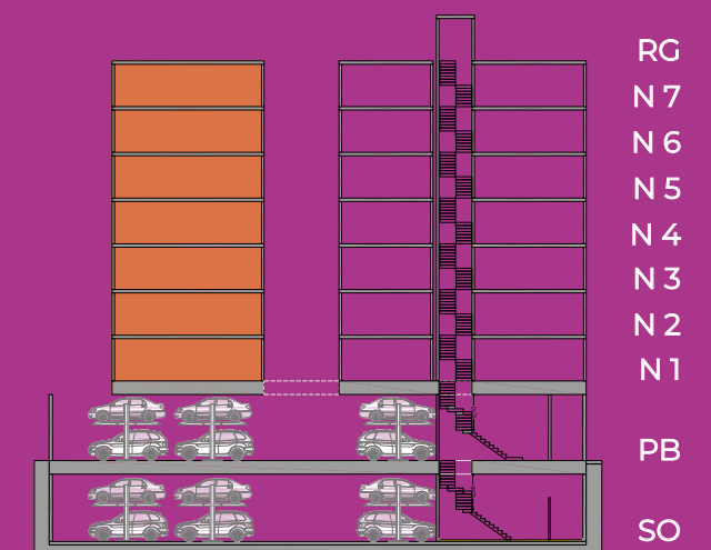
Sección esquemática
