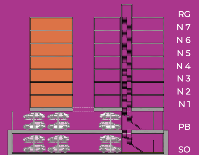
Sección esquemática
