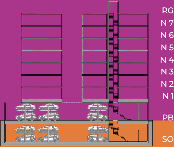
Sección esquemática
