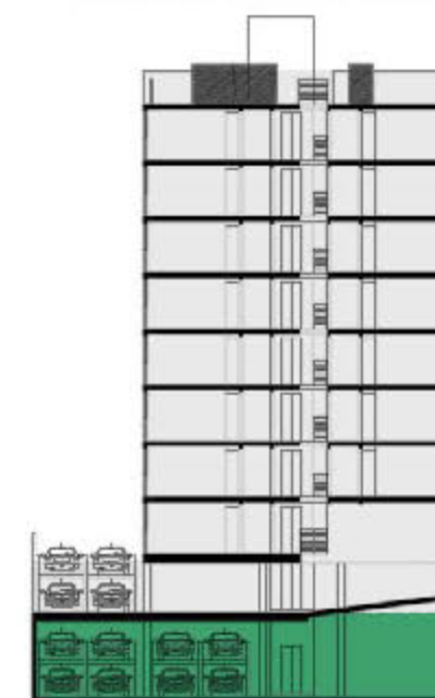
CORTE ESQUEMATICO
