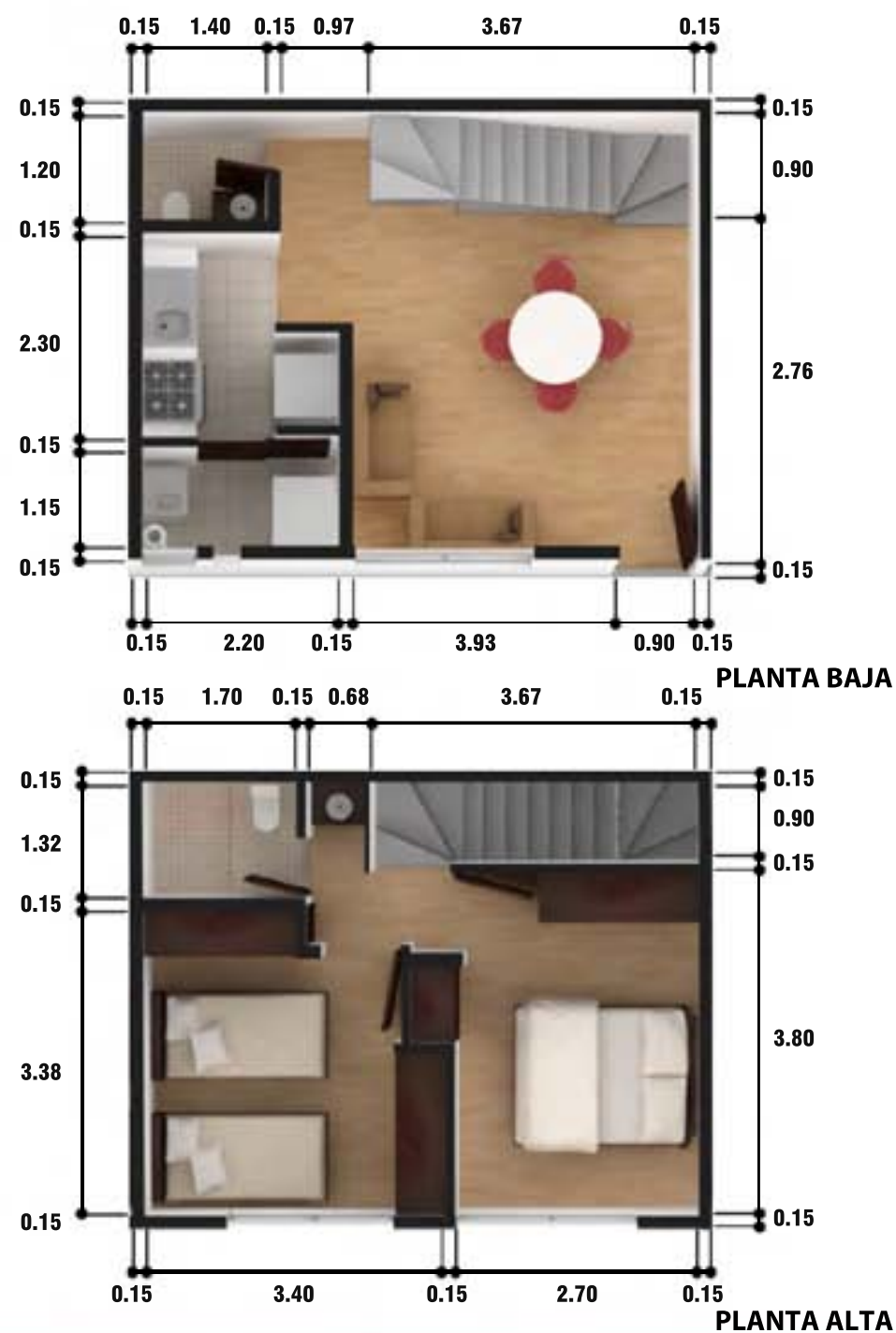
DEPARTAMENTO TIPO 9
