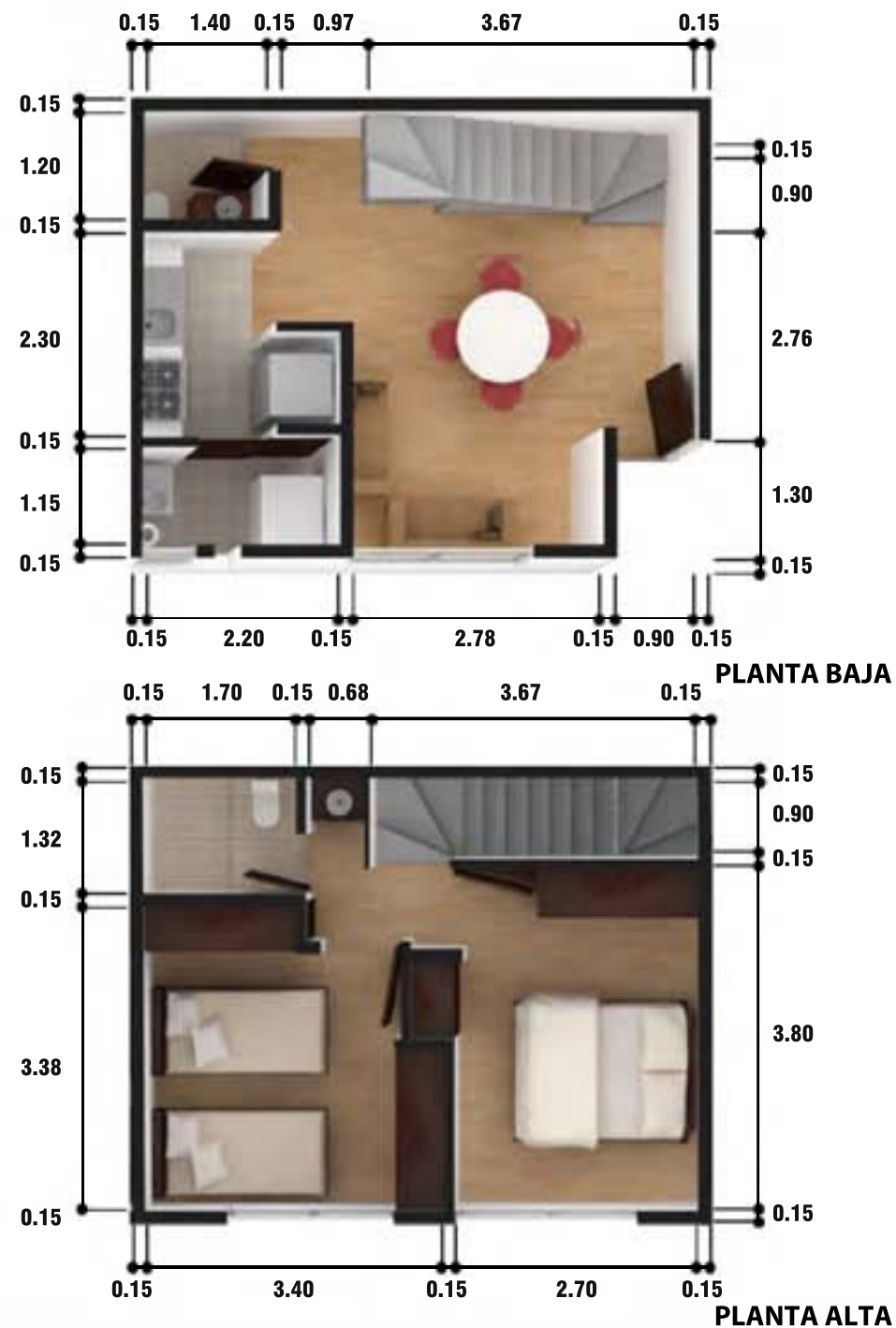
DEPARTAMENTO TIPO 8
