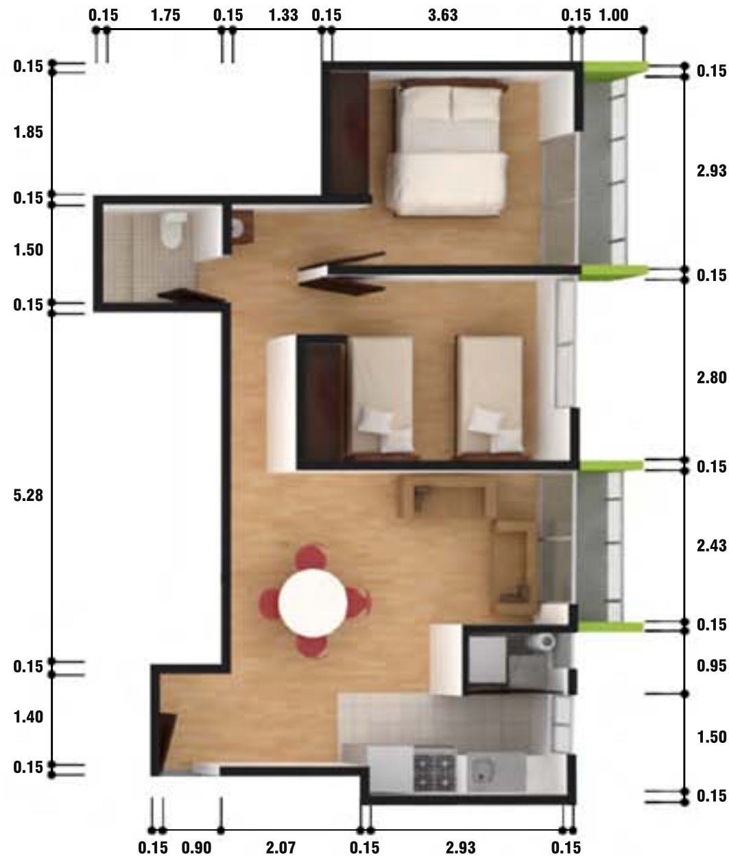
DEPARTAMENTO TIPO 2
